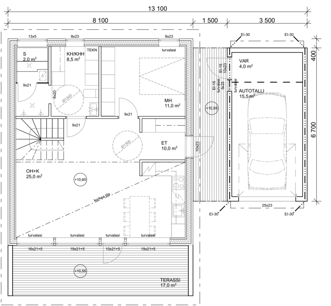
POHJAPIIRROS, 1.-KERROS
