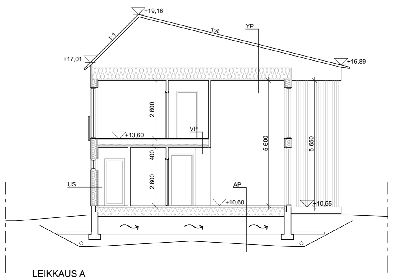
LEIKKAUS A
