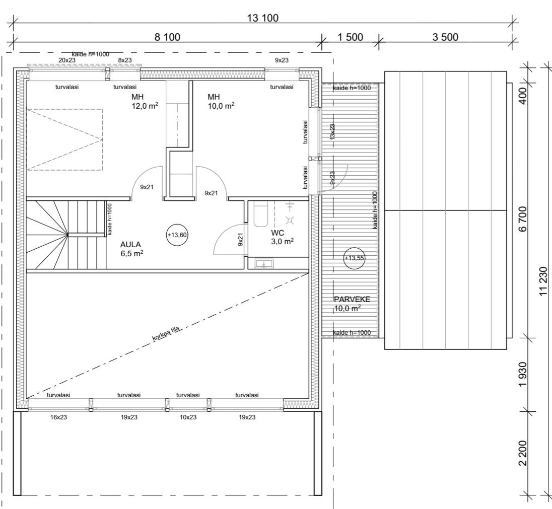
POHJAPIIRROS, 2.-KERROS
